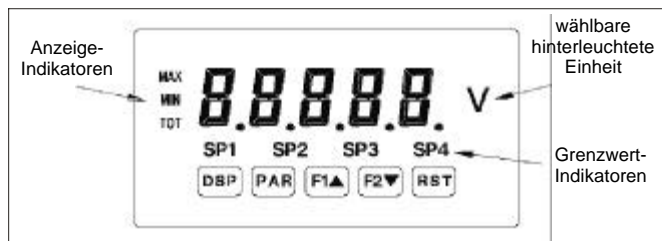
Frontansicht
