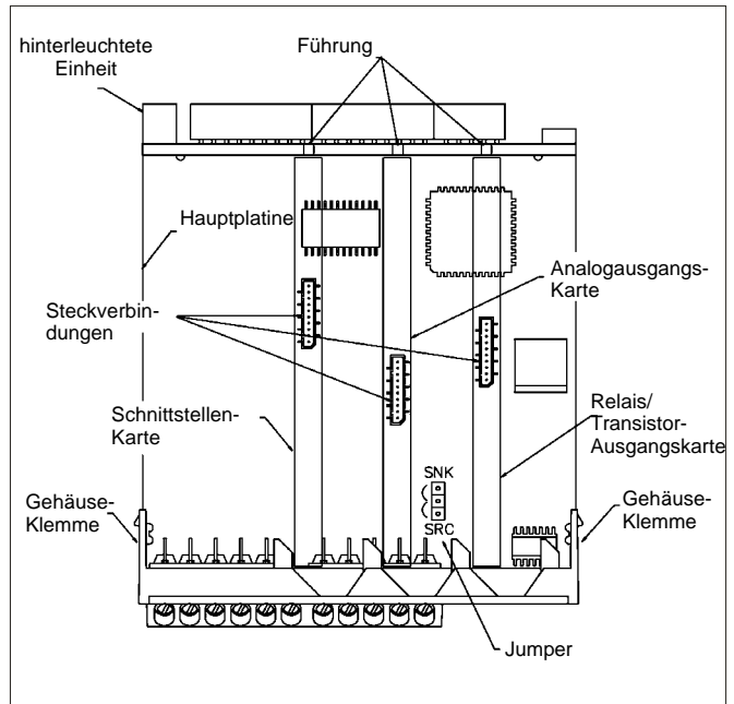
Mechanischer Aufbau
